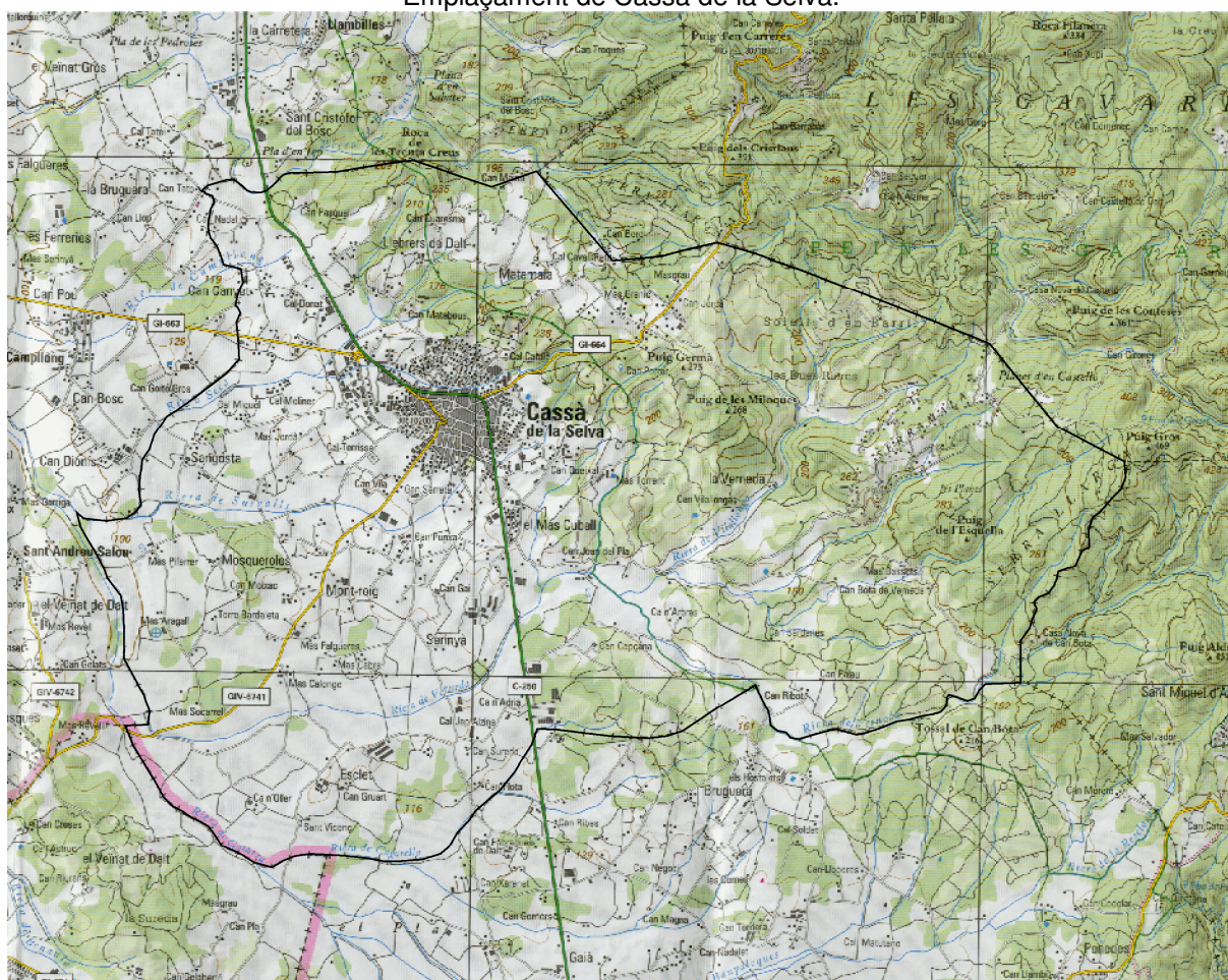
Figura 1.1.1. Emplaçament de Cassà de la Selva.
